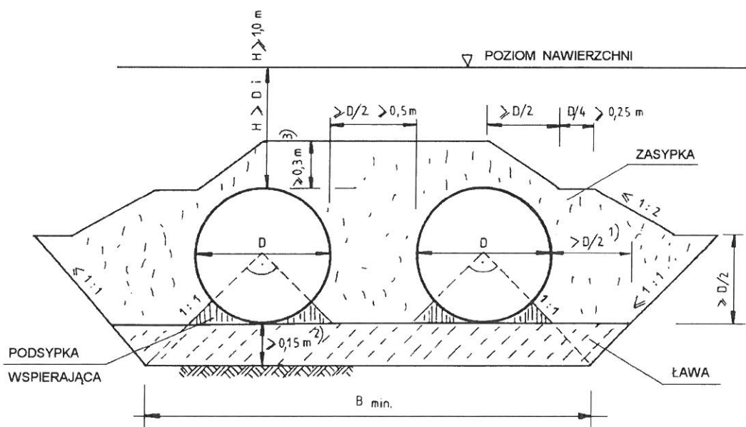
Rys. 8. Zasyпка nad przepustem dwururowym
