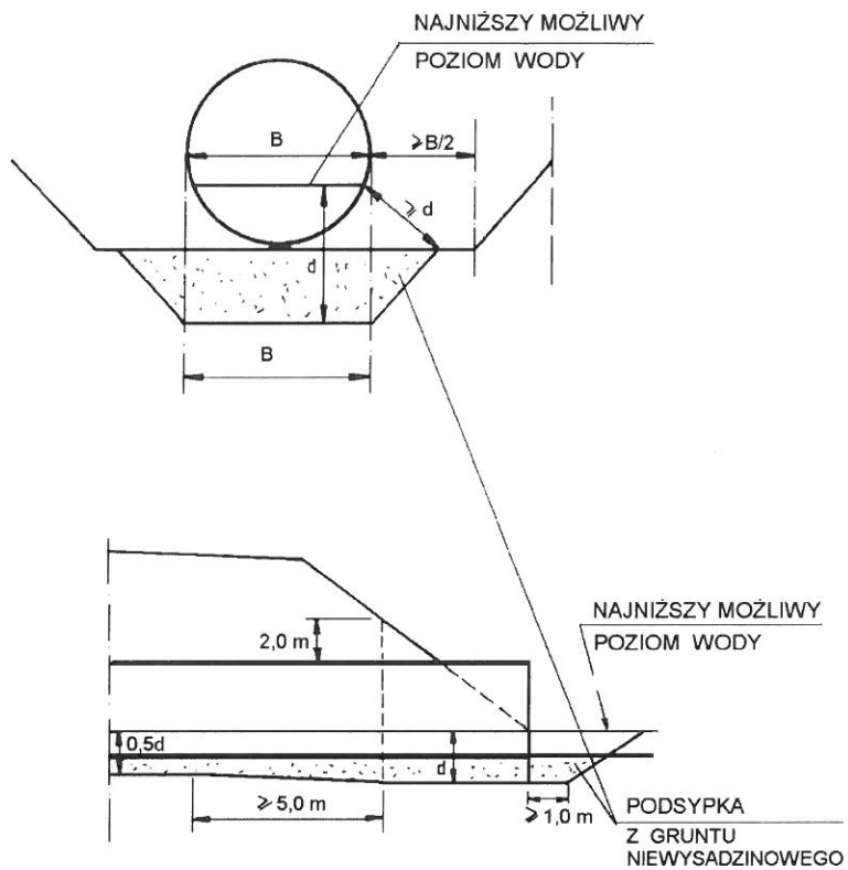
Rys. 6. Końcowy, skrajny odcinek rury nie powinien być krótszy od 1 m
