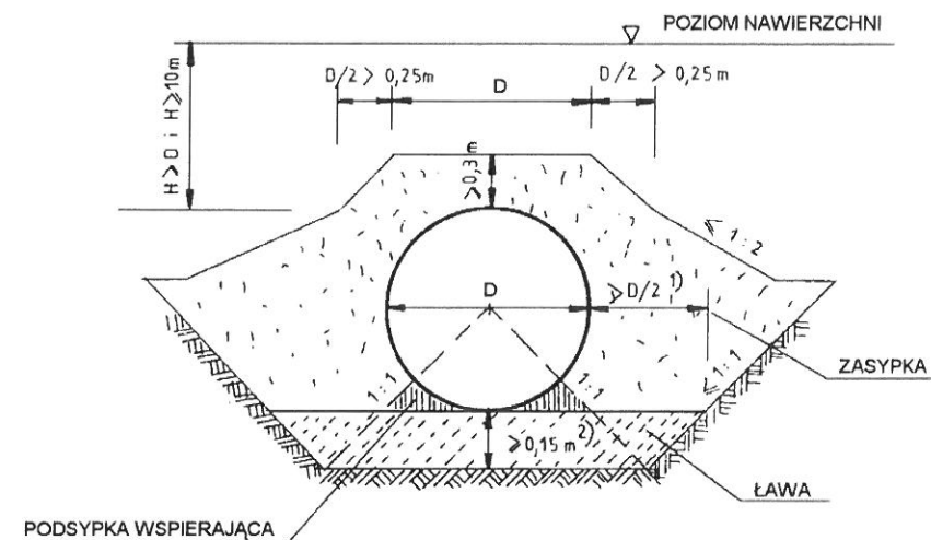
Rys. 7. Zasyпка nad przepustem jednorurowym
