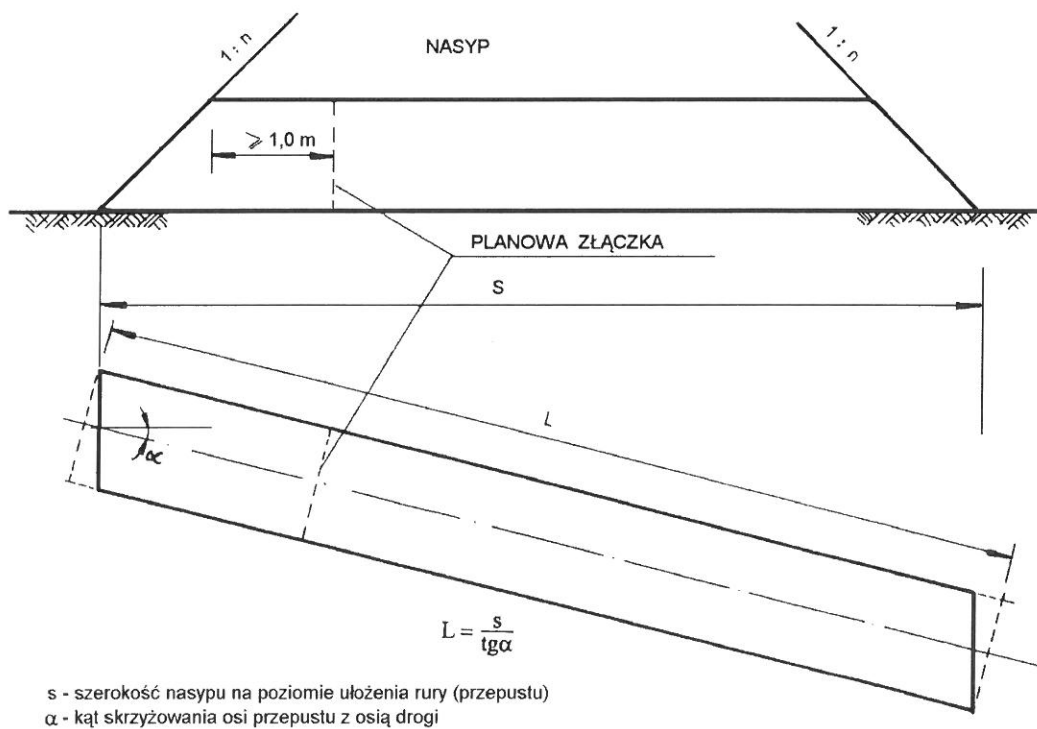
Rys. 6. Końcowy, skrajny odcinek rury nie powinien być krótszy od 1 m
