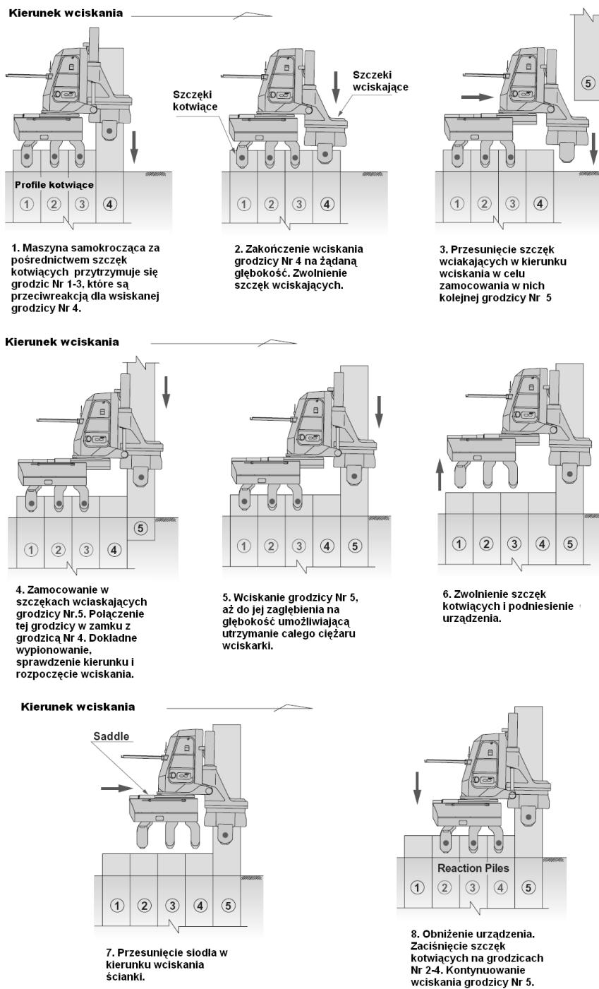
Rysunek 2. Procedura wciskania grodzic urządzeniem samokroczącym
