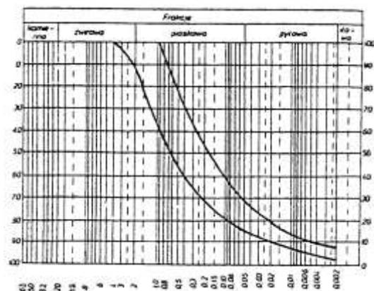
Rysunek 1. Obszar uziarnienia optymalnej mieszanki gliniasto-piaskowej
