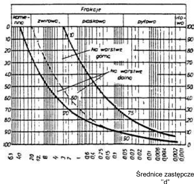
Rysunek 2. Obszar uziarnienia optymalnych mieszanek gliniasto-żwirowych
