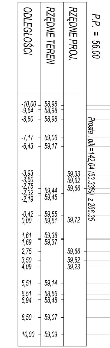
PK = 2+956,00 Skala 1:200/200
