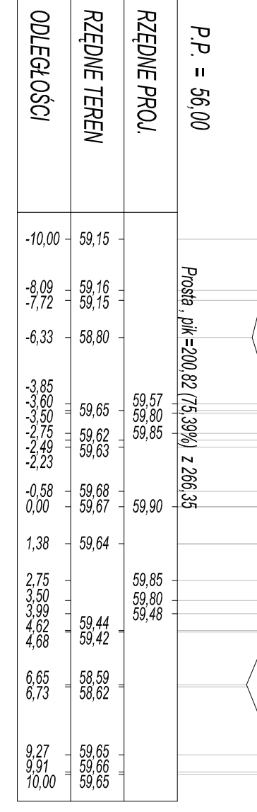
PK = 2+967,56 Skala 1:200/200
