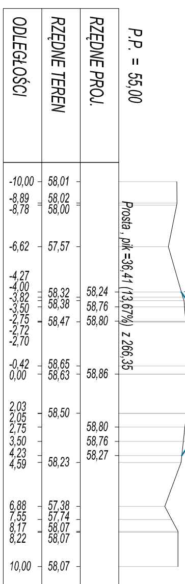
PK = 2+903,25 Skala 1:200/200
