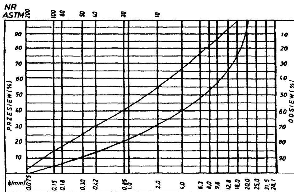
Rys. 9. Krzywe graniczne uziarnienia mieszanki mineralnej 0+16 mm do warstwy wiążącej, wyrównawczej i wzmocniającej z betonu asfaltowego dla KR 1-2
