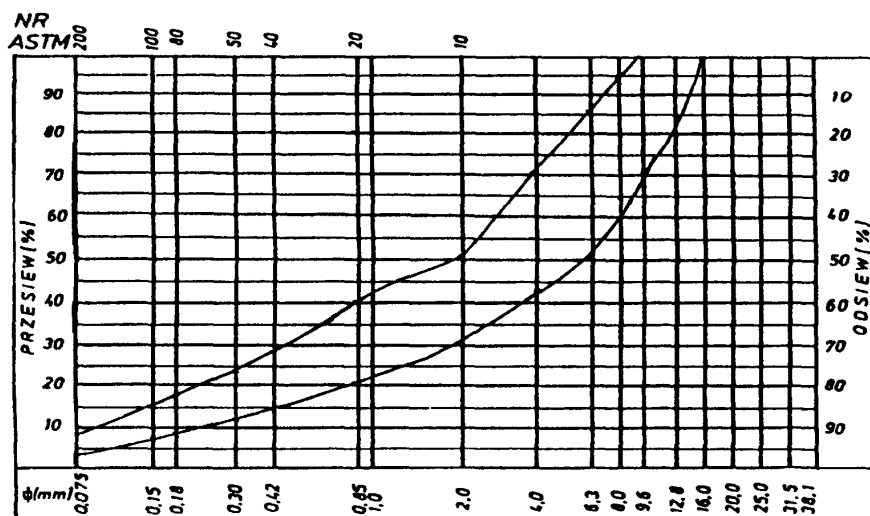
Rys. 8. Krzywe graniczne uziarnienia mieszanki mineralnej 0+20 mm do warstwy wiążącej, wyrównawczej i wzmocniającej z betonu asfaltowego dla KR 1-2
