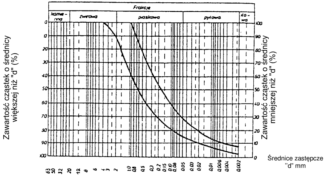
Rysunek 1. Obszar uziarnienia optymalnej mieszanki gliniasto-piaskowej
