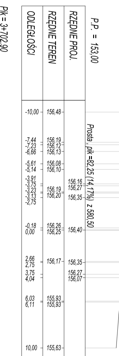
PK = 3+687,80 Skala 1:200/200
