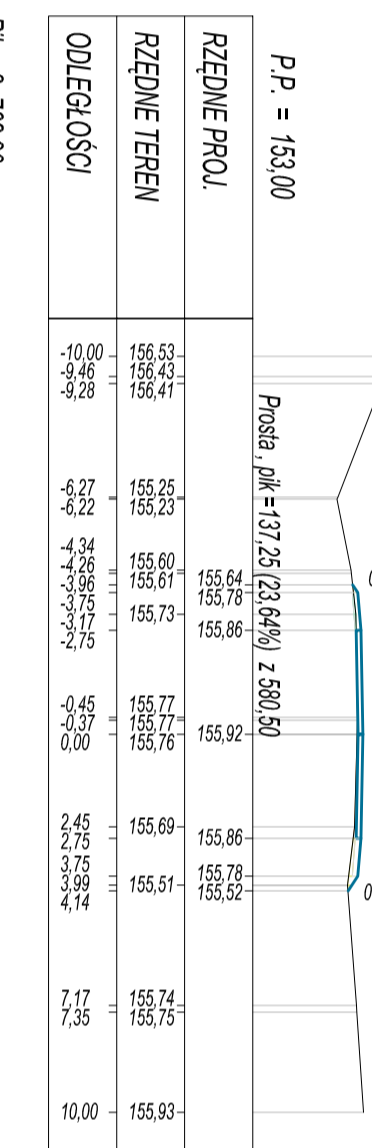
PK = 3+742,80 Skala 1:200/200
