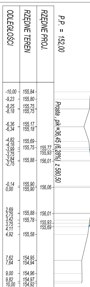
PK = 3+642,00 Skala 1:200/200
