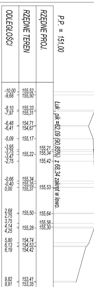
PK = 3+599,30 Skala 1:200/200
