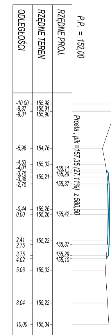
PK = 3+784,90 Skala 1:200/200
