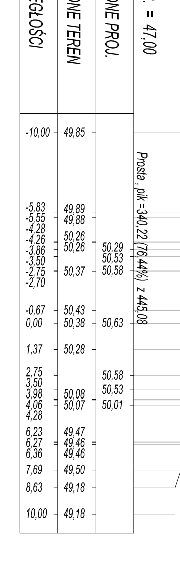
PK = 2+249,16 Skala 1:200/200
