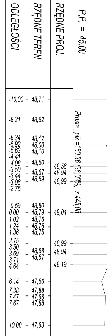
PK = 2+069,30 Skala 1:200/200
