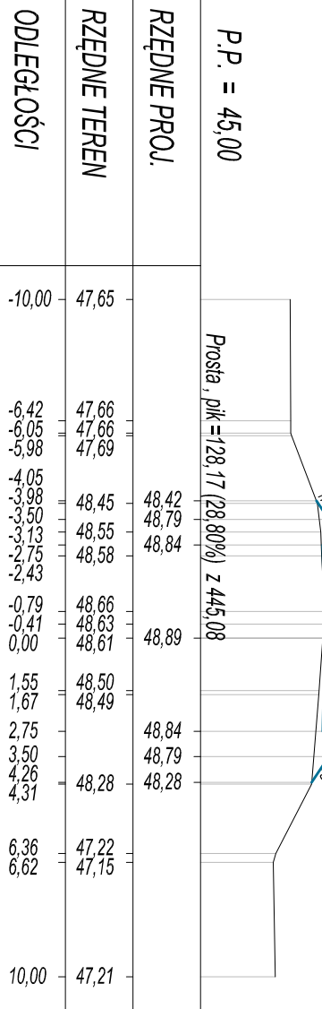
PK = 2+037,11 Skala 1:200/200
