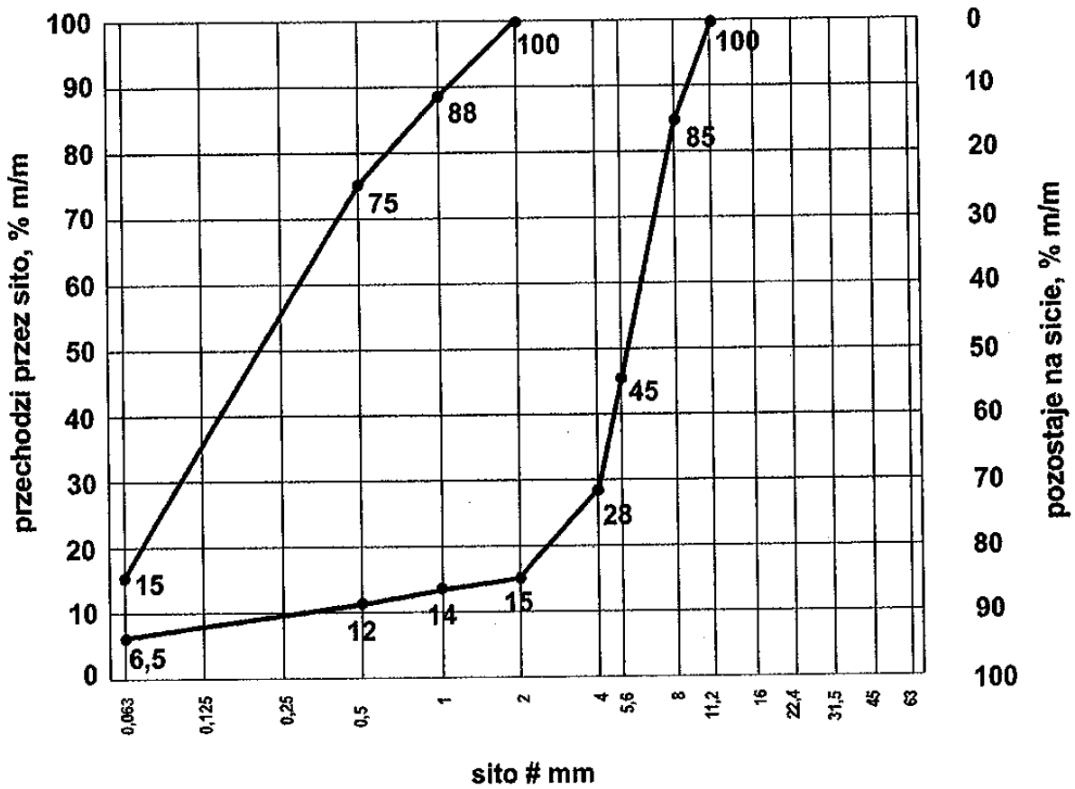
Rys. 4. Krzywe graniczne uziarnienia mieszanki mineralnej 0/11,2 mm
