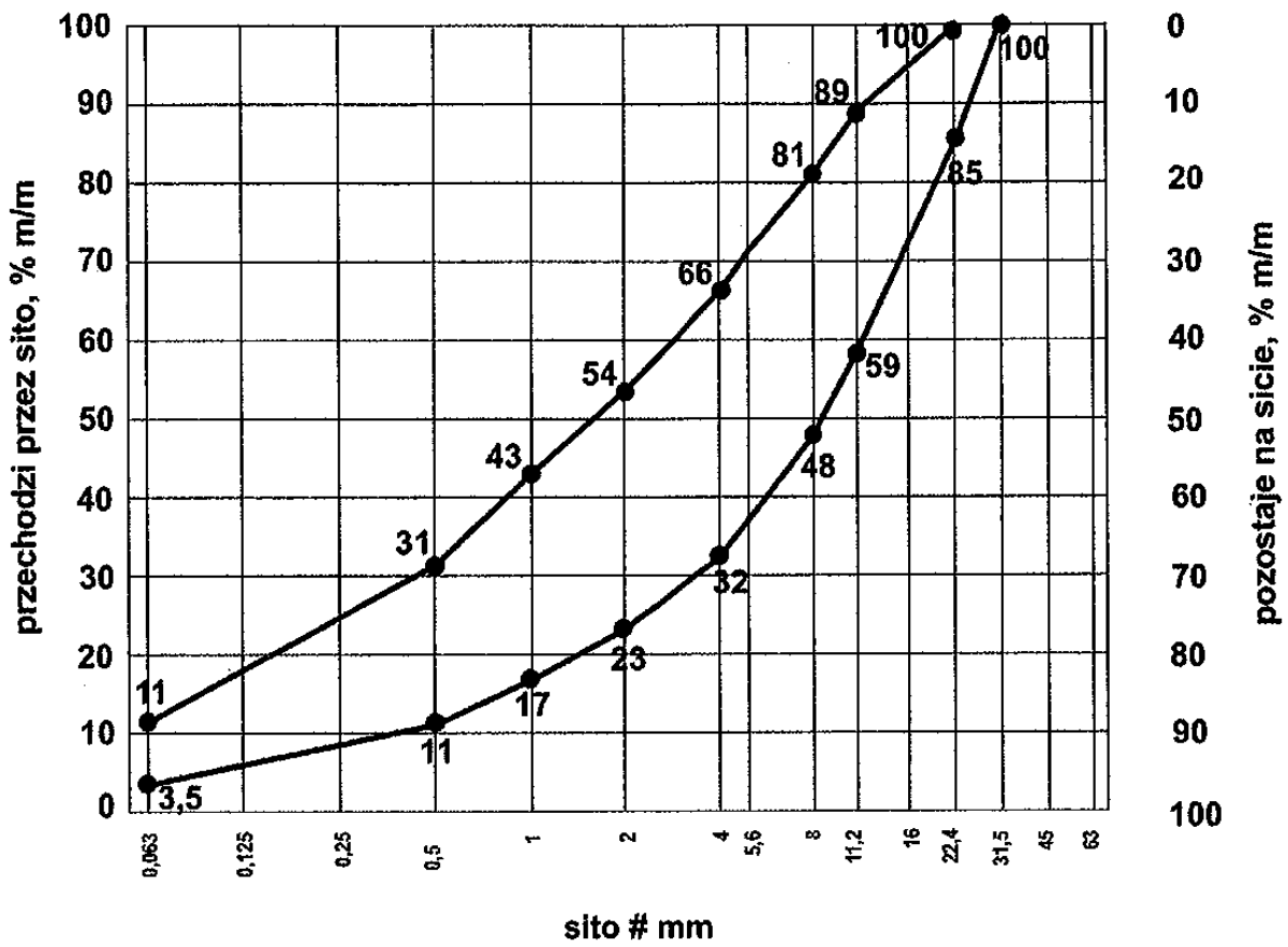
Rys. 2. Krzywe graniczne uziarnienia mieszanki mineralnej 0/22,4 mm
