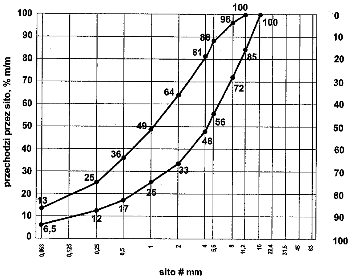
Rys. 4. Krzywe graniczne uziarnienia mieszanki mineralnej 0/11,2 mm
