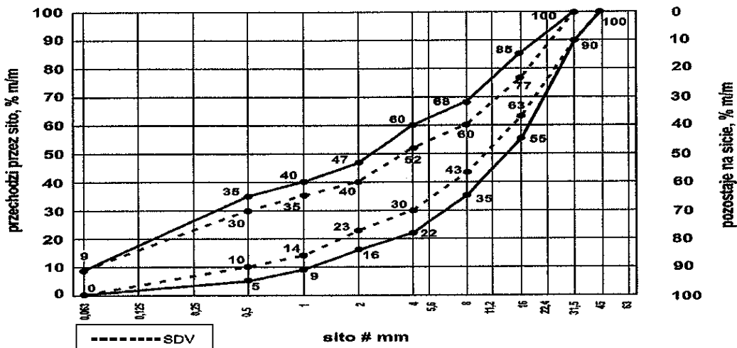
Rys. 1. Krzywe graniczne uziarnienia mieszanki kruszywa niezwiązanej 0/31,5 mm dla nawierzchni pobocza
