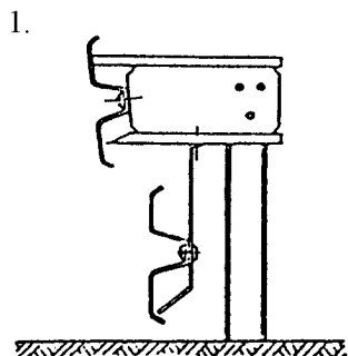
Załącznik 11.6. Sposoby lokalizowania barier w przekroju poprzecznym drogi, wg [32]
